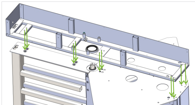
Рисунок 9.10 - Крепление корпуса механизма турникета
