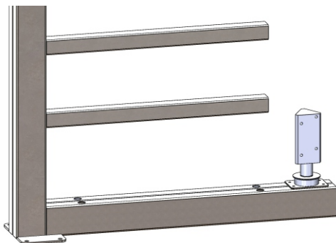
Рисунок 9.17 - Установленный нижний подшипниковый узел в модели без подогрева
