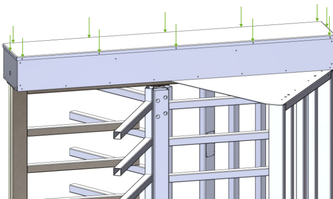
Рисунок 9.24 - Места крепления крышки корпуса механизма
