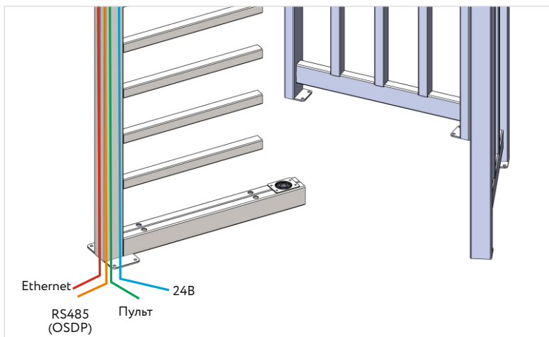
Рисунок 9.2 - Ввод кабелей в турникет 3V Model X / Xi
