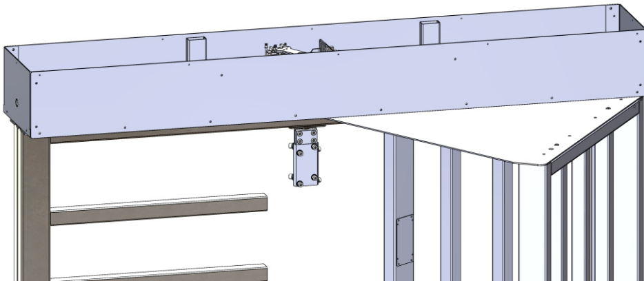
Рисунок 9.15 - Турникет с правильным положением верхнего подшипникового узла
