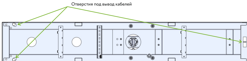
Рисунок 9.9 - Корпус механизма (вид сверху)
