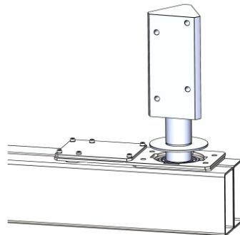
Рисунок 9.18 - Установленный нижний подшипниковый узел в модели с подогревом УХЛ 2.1
